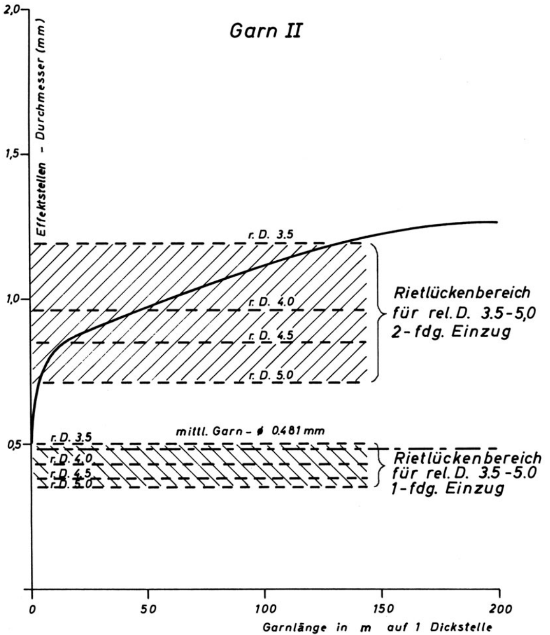
Abb. 6: Effektstellen-Durchmesser und ihre Häufigkeit in Zusammenhang mit Rietlücken und Gewebeeinstellungen
