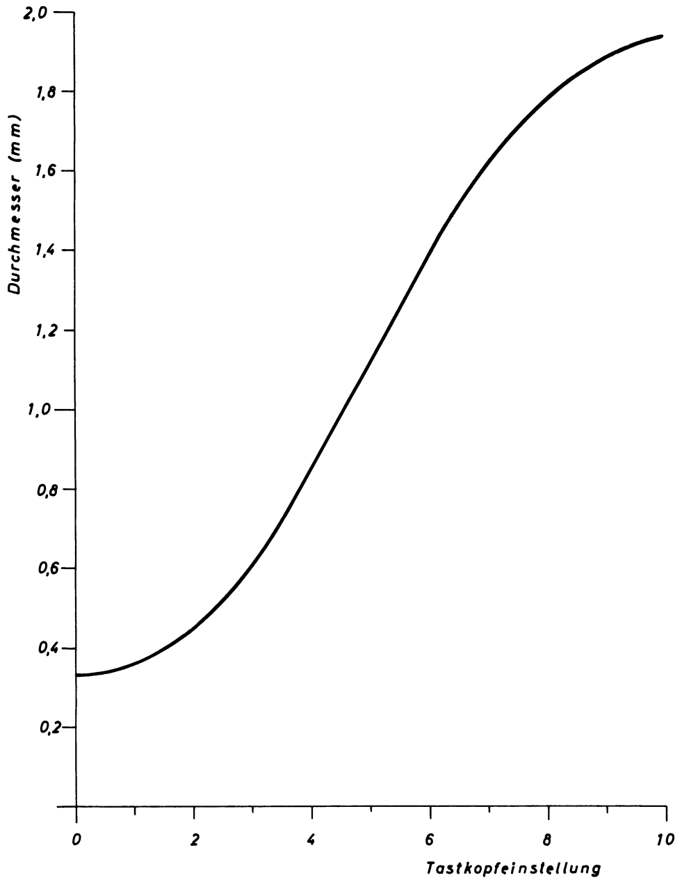
Abb. 1: Meßkopf-Eichkurve
