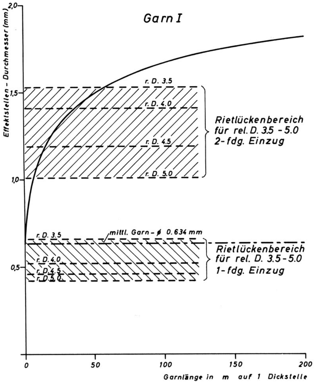
Abb. 5: Effektstellen-Durchmesser und ihre Häufigkeit in Zusammenhang mit Rietlücken und Gewebeeinstellungen
