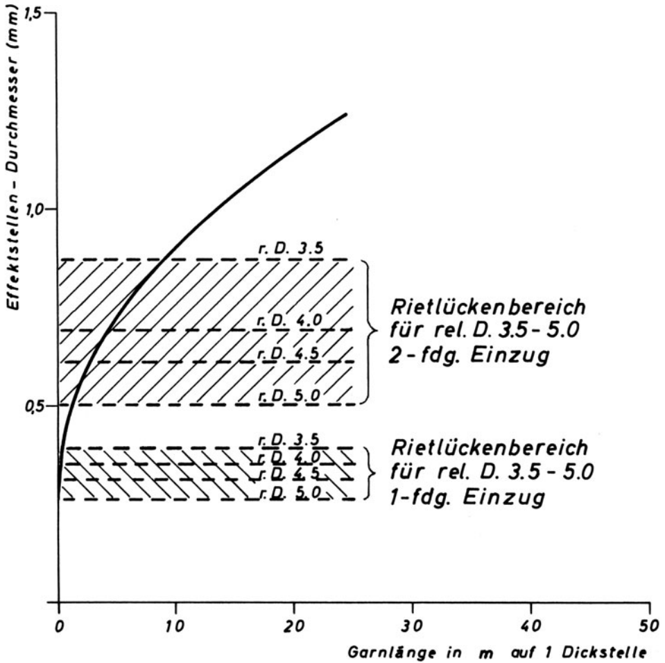
Abb. 7: Effektstellen-Durchmesser und ihre Häufigkeit in Zusammenhang mit Rietlücken und Gewebeeinstellungen
