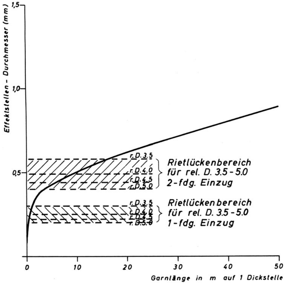
Abb. 8: Effektstellen-Durchmesser und ihre Häufigkeit in Zusammenhang mit Rietlücken und Gewebeeinstellungen
