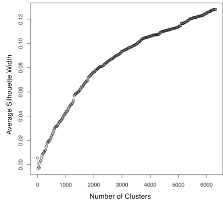
(d) FSM+Dependency
