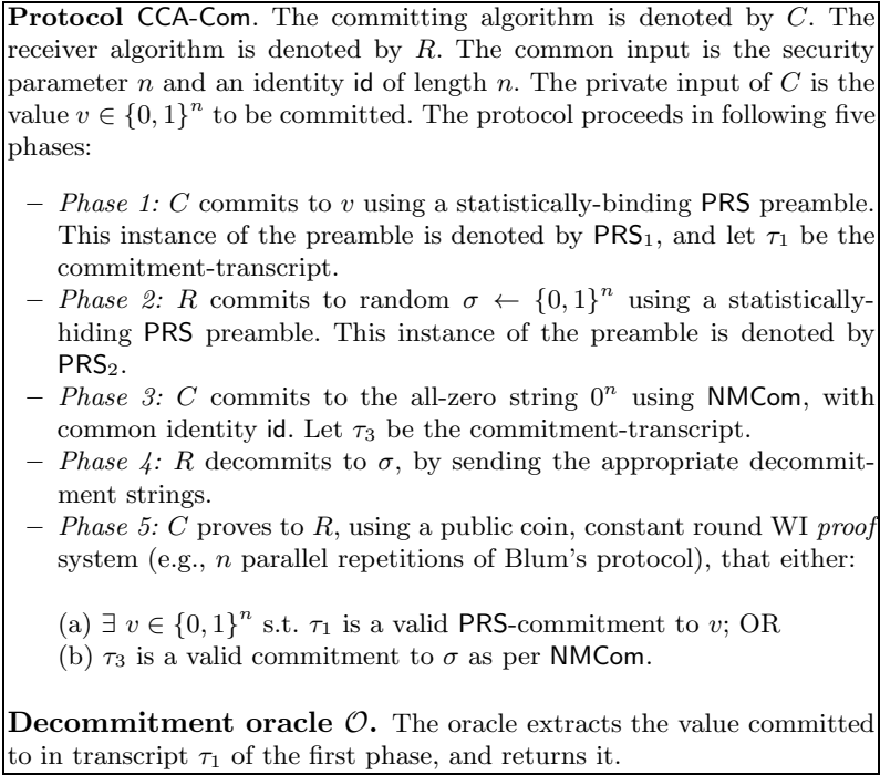
Fig. 3. Protocol CCA-Com
