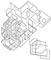
Abb. 62. Salpetersaurer Harnstoff.
