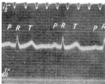
Abb. 36. Normales Elektrokardiogramm.
