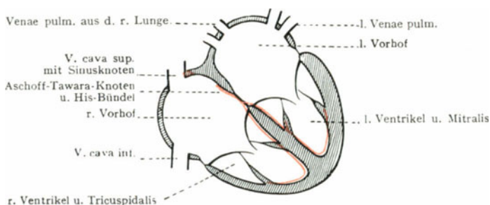
Abb. 26. Schematische Darstellung des Sinusknotens von Keith und Flack sowie des Aschoff-Tawaraschen Knotens im Septum der Vorhöfe wie des davon ausgehenden Hischen-Bündels zu den Papillarmuskeln und zu der Wand beider Ventrikel.
