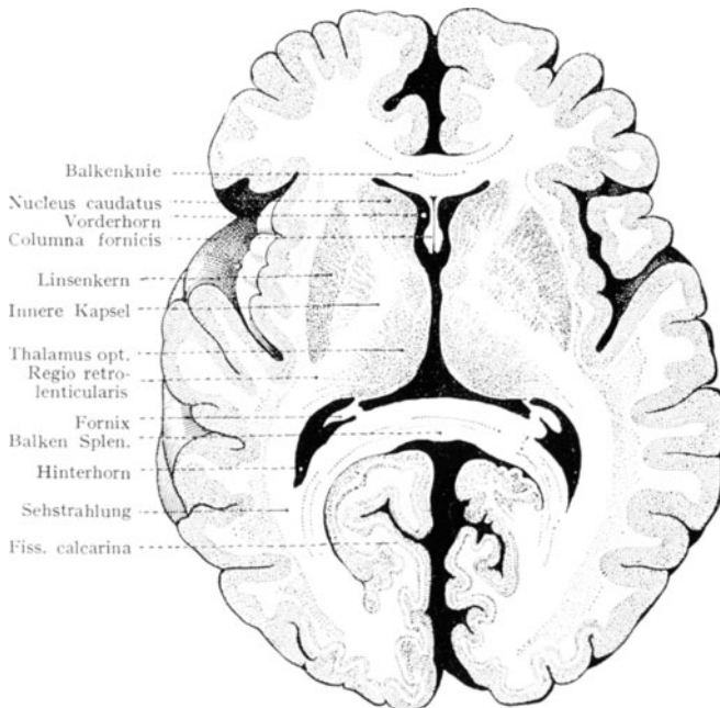
Abb. 122. Horizontalschnitt durch das Großhirn.
