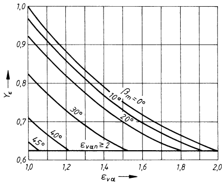
TB 22-3 Überdeckungsfaktor (Zahnfuß) Y_e für \alpha_n = 20^\circ (nach DIN 3991 T3)
