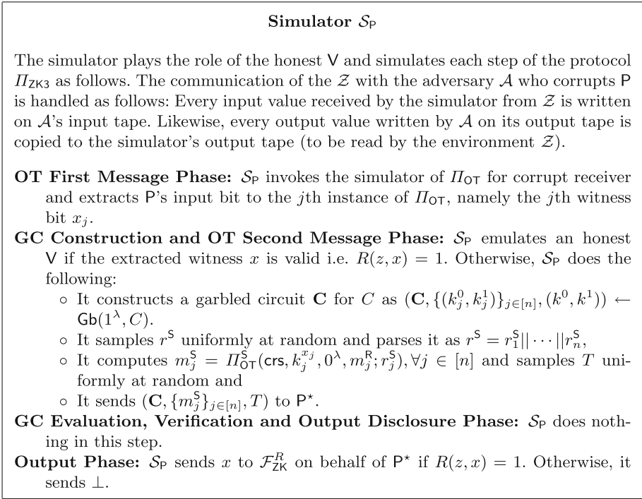
Fig. 4. Simulator \mathcal{S}_P
