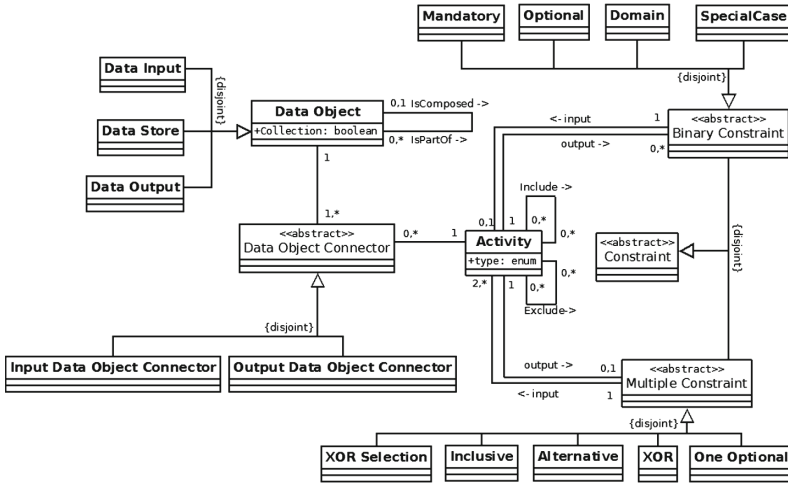
Fig. 5. BPFM meta-model
