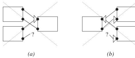
Fig. 3. Forbidden DAAs
